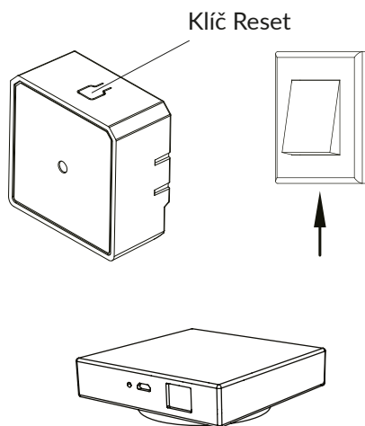
Brána Zigbee
